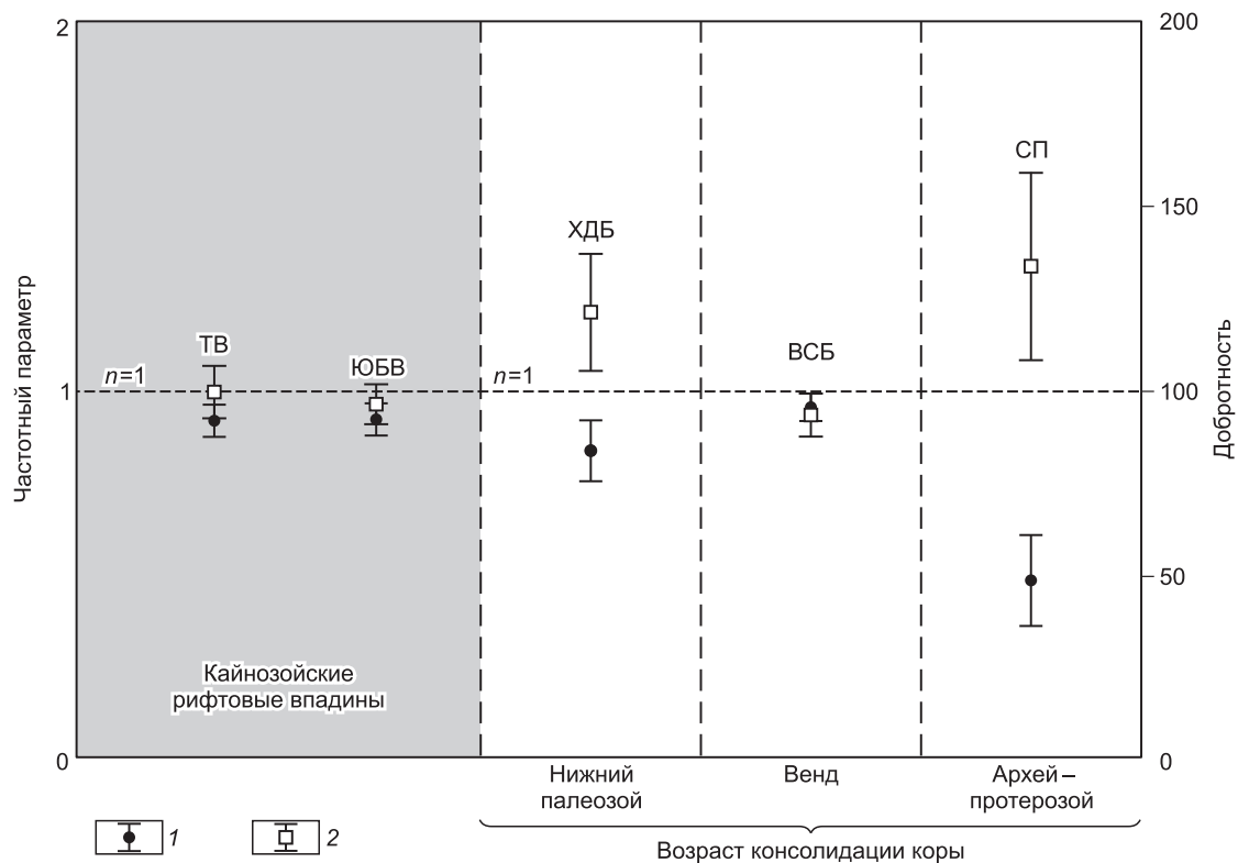
Рис. 6. Частотный параметр ( n ) и добротность ( Q_0 ) для отдельных сегментов рассматриваемой территории.
