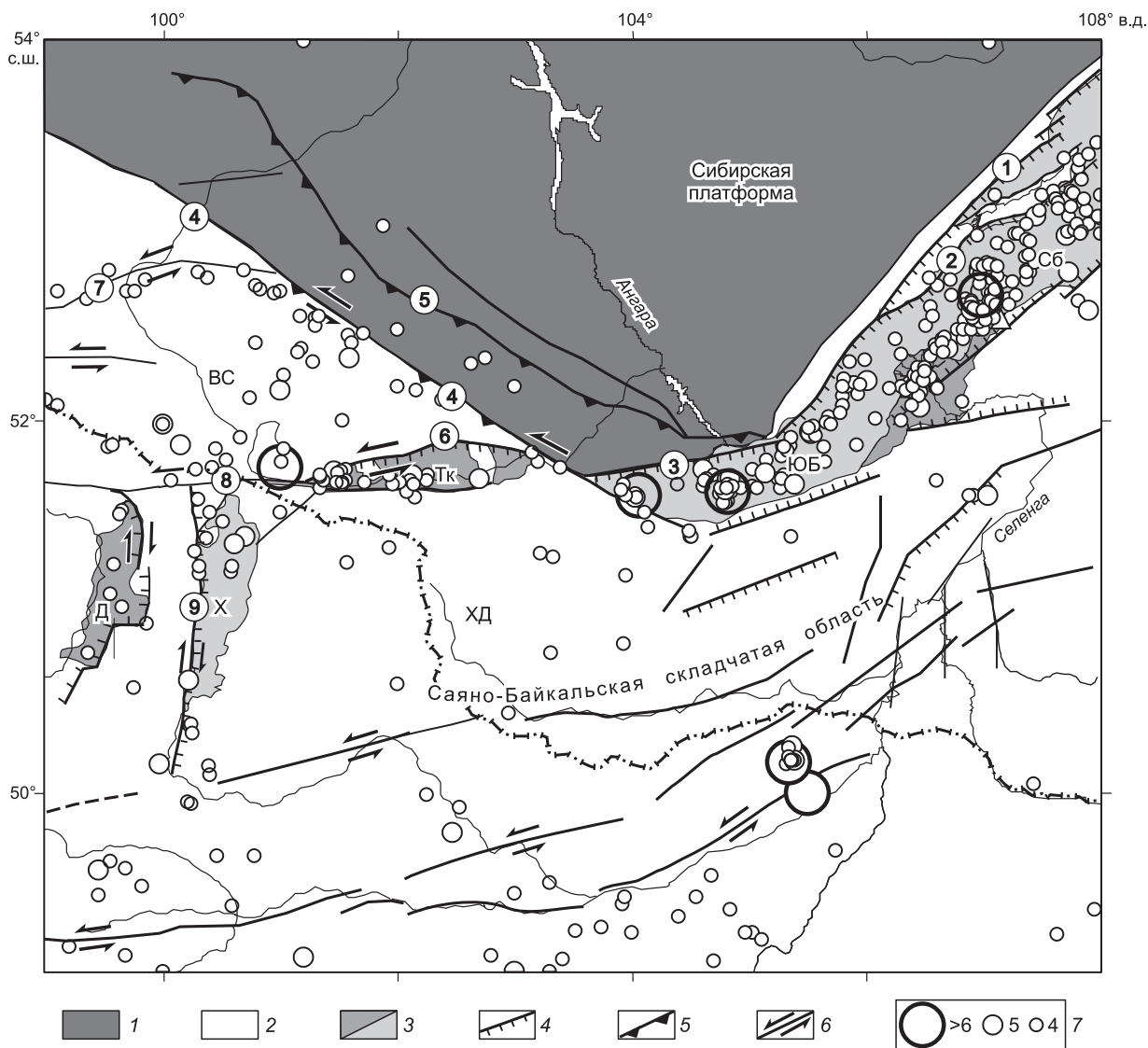
Рис. 1. Схема неотектонических структур и сейсмичность юго-западного фланга Байкальской рифтовой системы и его окружения.
