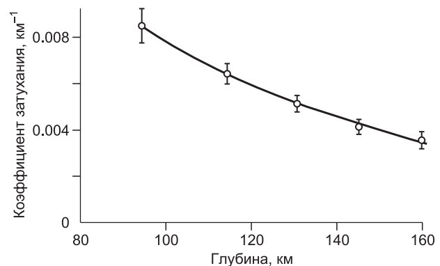
Рис. 5. Зависимость коэффициента затухания ( \delta ) от глубины нижней границы эллипсоида ( c ).
